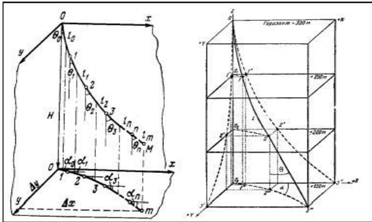
Рис. Викривлення свердловин: I — загальний вигляд в аксонометричній проекції; 1, 2, 3 — просторове положення вісі свердловини; I', 2', 3' — профіль вісі викривленої свердловини в проекції на координатну площину YOZ; I'', 2'', 3'' — профіль вісі викривленої свердловини в проекції на координатну площину XOZ; I''', 2''', 3''' — проекція вісі свердловини на горизонтальну площину плану XOY; II — схема інклінометричної зйомки викривлення свердловини; O, o — відповідно устя свердловини та його проекція на горизонтальну площину плану; M — відповідно вибій свердловини та його проекція на горизонтальну площину плану; 0, 1, 2, 3... n — точки виміру викривлення свердловини при інклінометричній зйомці; l_0, l_1, l_2 \dots l_n — відстані (інтервали) вздовж вісі свердловини між точками виміру викривлення; \alpha_i, \theta_i — відповідно дирекційний та зенітний кути i-го інтервалу; \Delta X, \Delta Y — відповідно приращення координат X і Y між проекціями устя та вибою свердловини.
