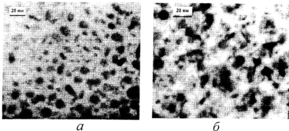
Рис. 4. ПЭМ-изображения мезоморфных стеклообразных композитов на основе каприлата кадмия с гетеронаночастицами CdSe/CdS (а) и CdS/CdSe (б).
