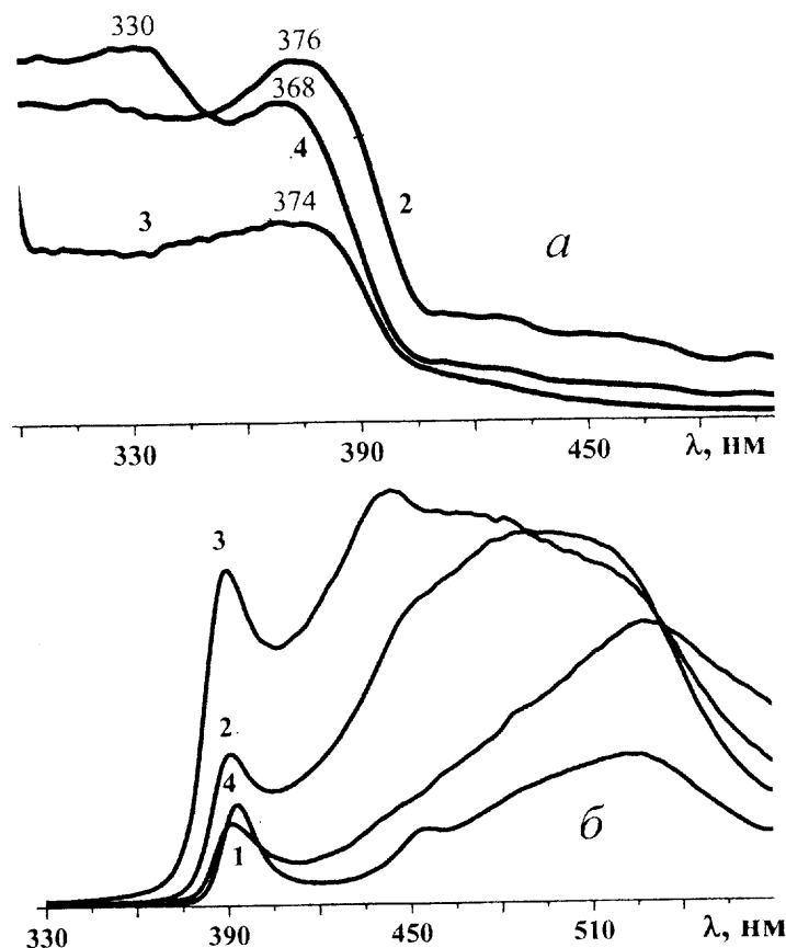
Рис. 6. Спектры возбуждения (а) и флуоресценции (б) стеклообразных мезоморфных нанокompозитов на основе каприлата кадмия с наночастицами CdSe (1) и гетеронаночастицами CdSe/CdS в зависимости от мольного соотношения S/Se: 2 — 3/1; 3 — 2/1; 4 — 1/3.
