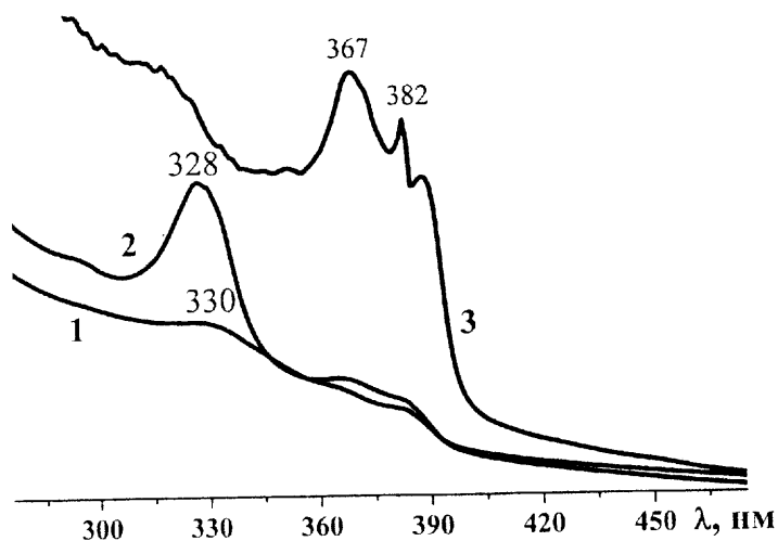
Рис. 5. Спектры поглощения стеклообразных мезоморфных нанокompозитов на основе каприлата кадмия с гетеронаночастицами CdSe/CdS в зависимости от мольного соотношения S/Se: 1 — 3/1; 2 — 2/1; 3 — 1/3. Здесь и на рис. 6 общая концентрация халькогенид-ионов — 4 % мол.
